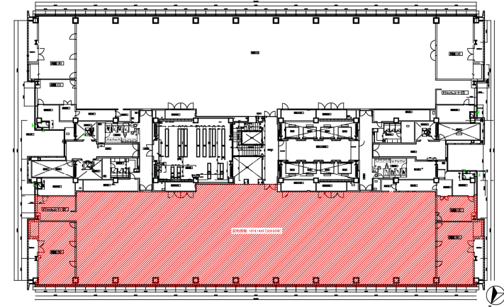
トレードピアお台場 【17F平面詳細図】17F
