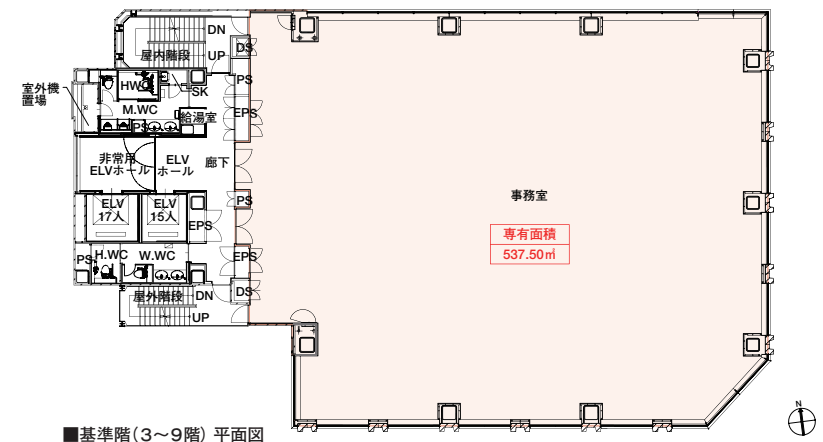
■基準階(3～9階) 平面図
