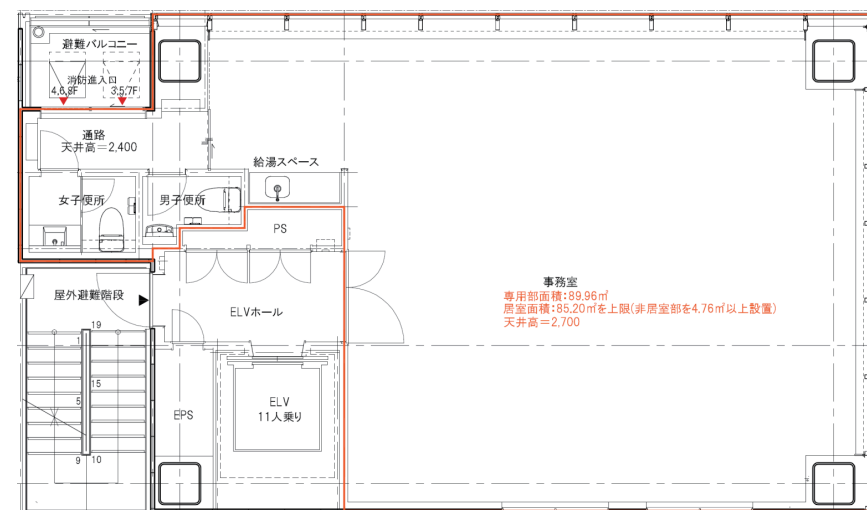
■基準階平面図(3~8階)
